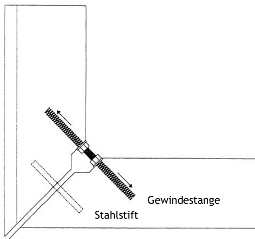
Eckverbindung
