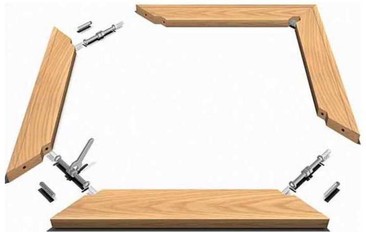
Regulierungssystem über Gewindebolzen und Mutter
